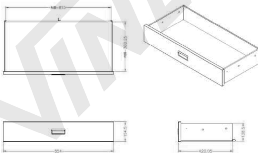
Dimensioni e proiezione n. 2 cassetti dim. cm 81,5 x 39,8 x 15,5 H
