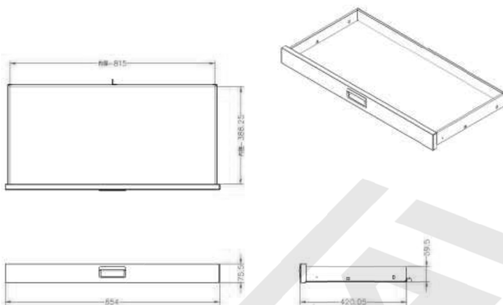
Dimensioni e proiezione n. 2 cassetti dim. cm 81,5 x 39,8 x 7,5 H
